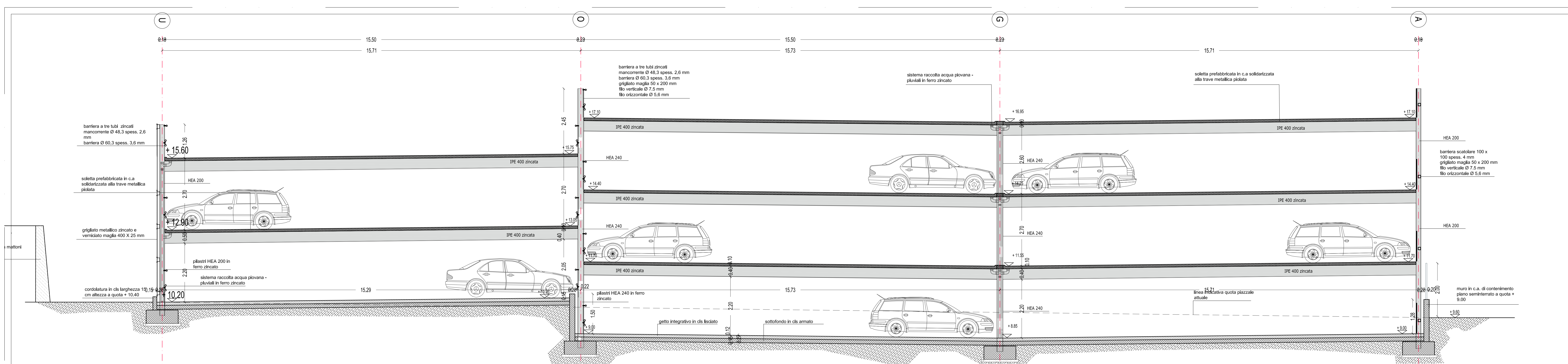
SEZIONE TRASVERSALE TIPO
