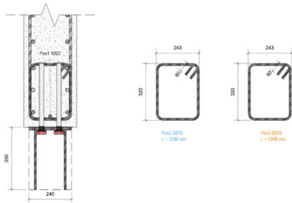
Sezione B-B
